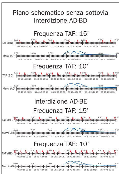
fig. 9 – Leggi di distribuzione degli arrivi su scala oraria. Piano di stazione senza sottovia
