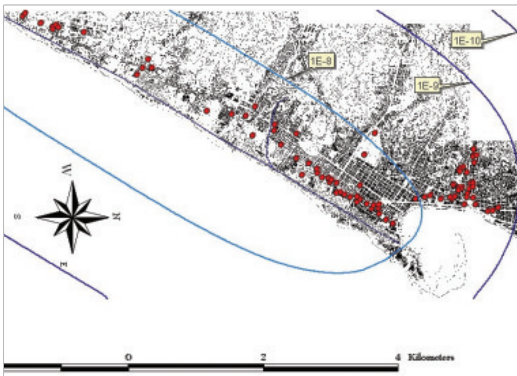
fig. 8 – Rischio locale dovuto al trasporto di sostanze pericolose nella rete ferroviaria nell'area di Messina
