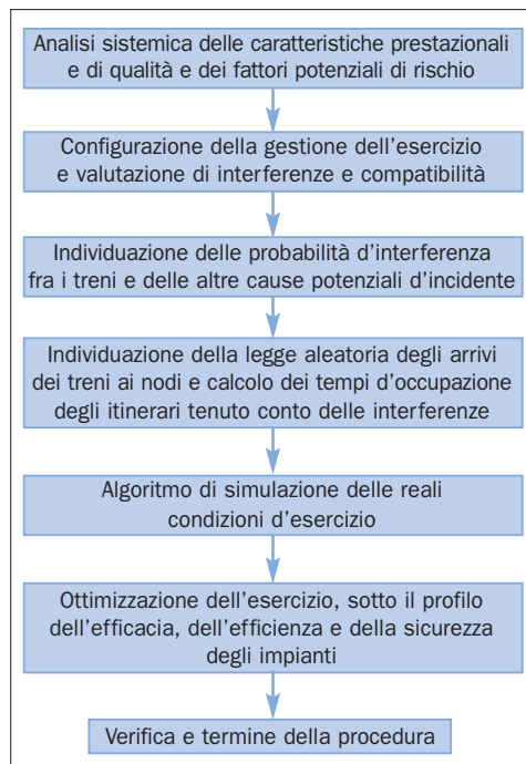
fig. 2 – Fasi logiche della metodologia d'approccio allo studio d'ottimizzazione
